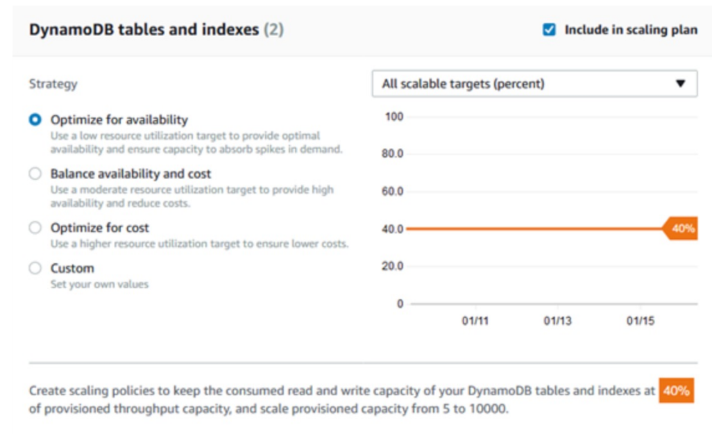
DynamoDB Tables
